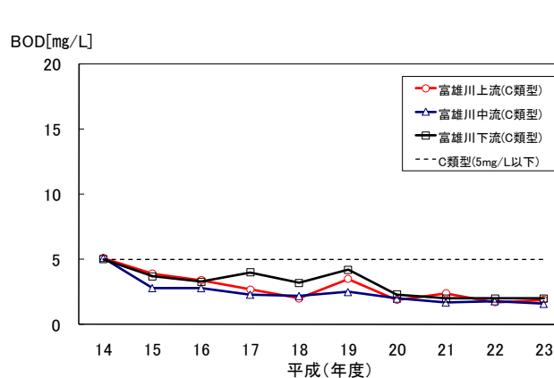
(図3-4-22) 富雄川のBOD推移 (75%値)
