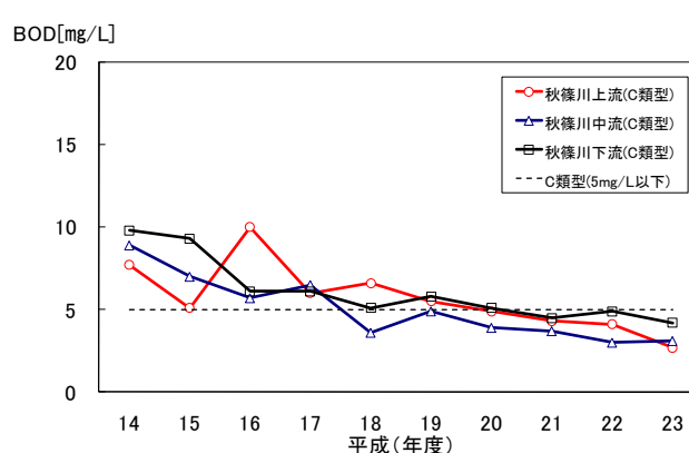
(図3-4-21) 秋篠川のBOD推移 (75%値)
