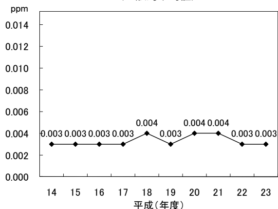
(図3-4-1) 二酸化硫黄濃度の経年変化 (一般局平均値)
