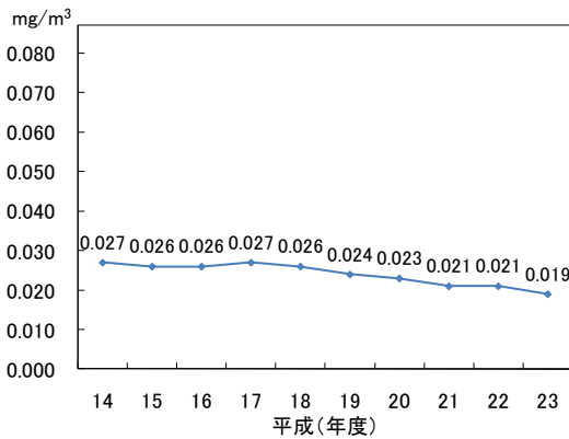
(図3-4-10) 浮遊粒子状物質濃度の経年変化 (一般局平均値)
