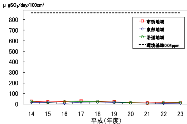
(図3-4-15) 硫黄酸化物の経年変化
