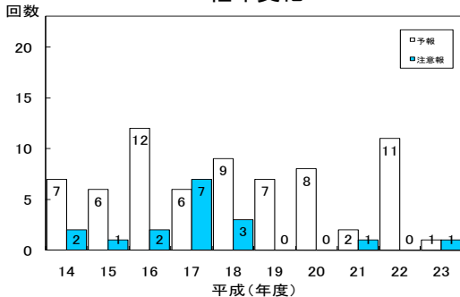
(図3-4-9) 光化学スモッグ発令回数 経年変化
