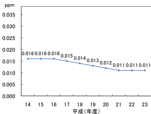
(図3-4-3) 二酸化窒素濃度の経年変化 (一般局平均値)
