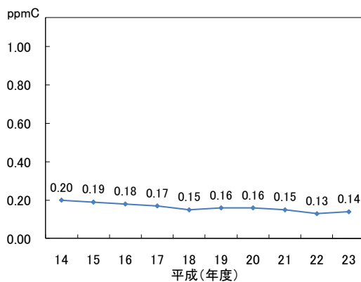
(図3-4-12) 非メタン炭化水素濃度の経年変化 (年平均値)
