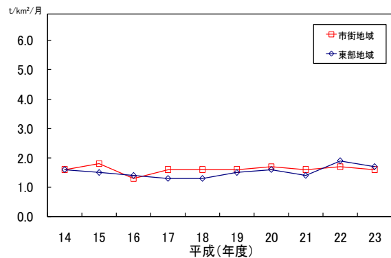
(図3-4-14) 降下ばいじんの経年変化
