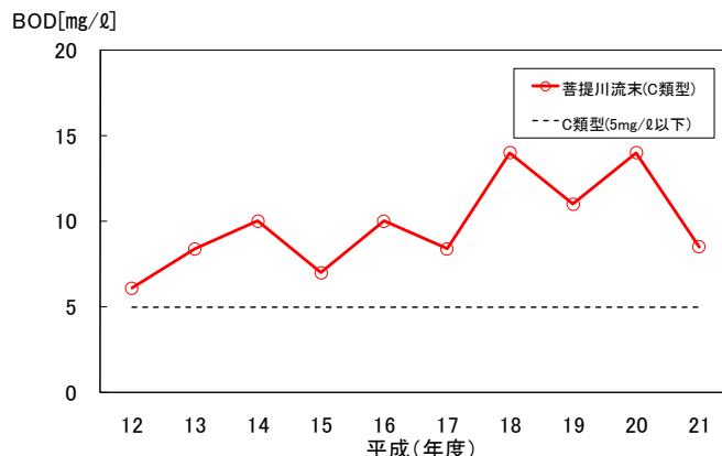
(図-2, 22) 菩提川のBOD推移 (75%値)
