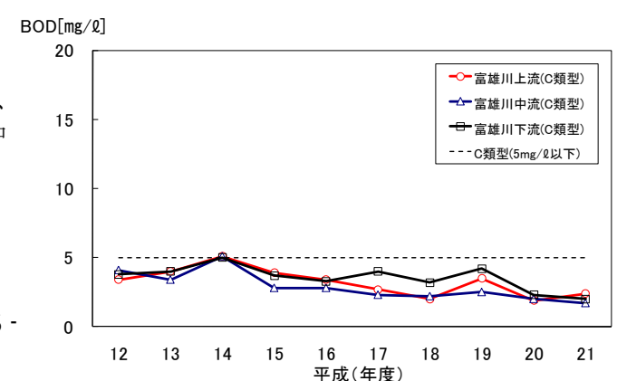
(図-2, 21) 富雄川のBOD推移 (75%値)
