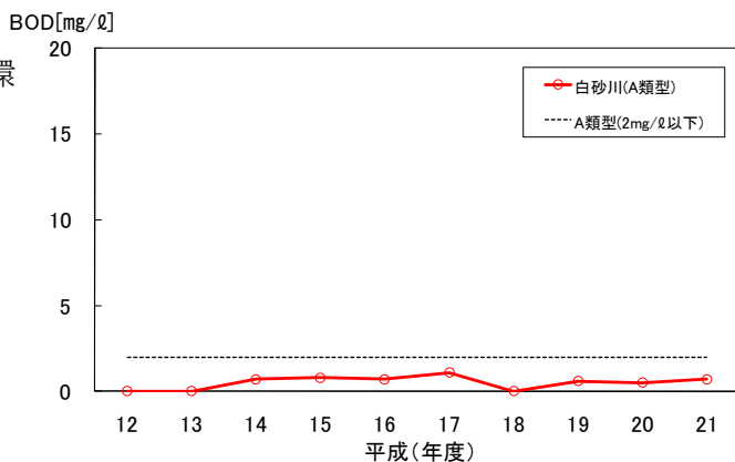
(図-2, 24) 白砂川のBOD推移 (75%値)
