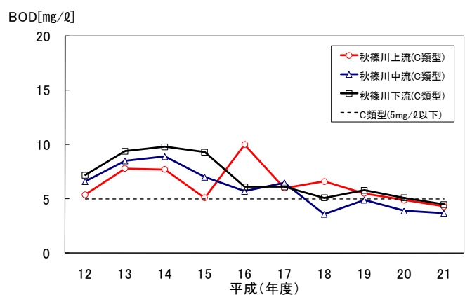
(図-2, 20) 秋篠川のBOD推移 (75%値)
