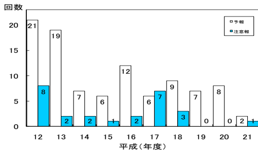
(図-2, 9) 光化学スモッグ発令回数の 経年変化 (表-2, 19) 光化学スモッグ発令区分と発令基準
