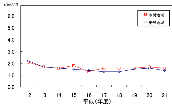
(図-2, 14) 降下ばいじんの経年変化
