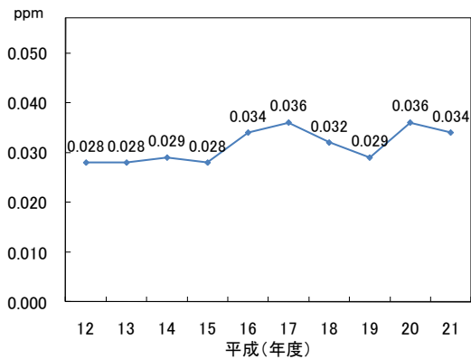
(図-2, 7) 光化学オキシダント濃度の 経年変化 (昼間の1時間値の年平均値)
