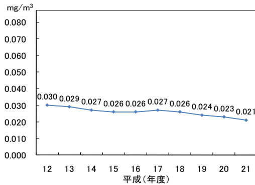
(図-2, 10) 浮遊粒子状物質濃度の 経年変化 (一般局平均値)
