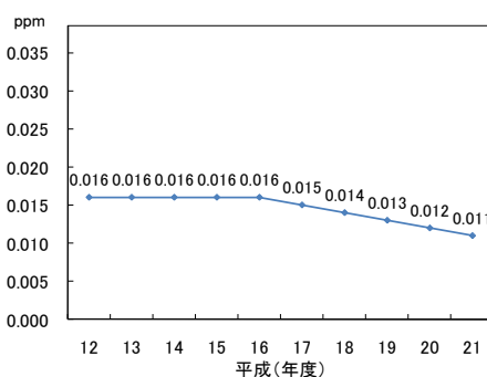
一般局平均値の経年変化
