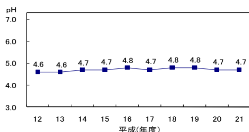
酸性雨の経年変化
