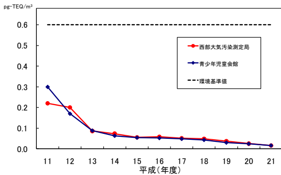
大気調査結果（経年変化） 単位：pg-TEQ/m 3
