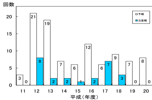
(図-2, 9) 光化学スモッグ発令回数 の経年変化
