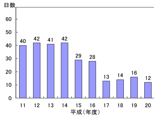
(図-2, 13) 非メタン炭化水素 (6-9時 3時間平均値が0.31ppmCを超えた日数)
