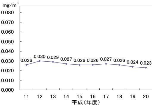
(図-2, 10) 浮遊粒子状物質濃度の 経年変化 (一般局平均値)
