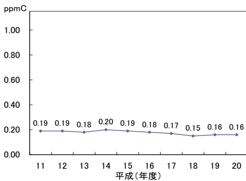
(図-2, 12) 非メタン炭化水素濃度の 経年変化 (年平均値)
