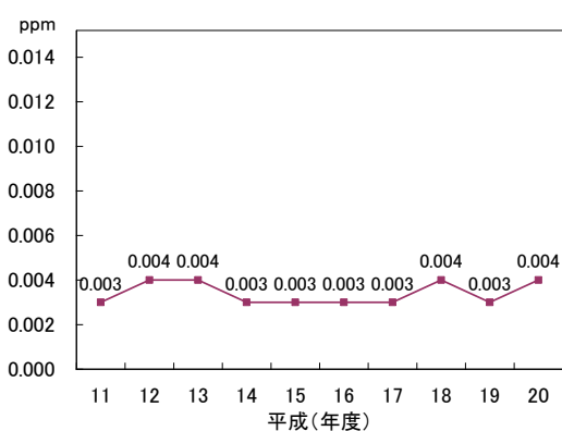
(図-2, 1) 二酸化硫黄濃度の経年変化 (一般局平均値)
