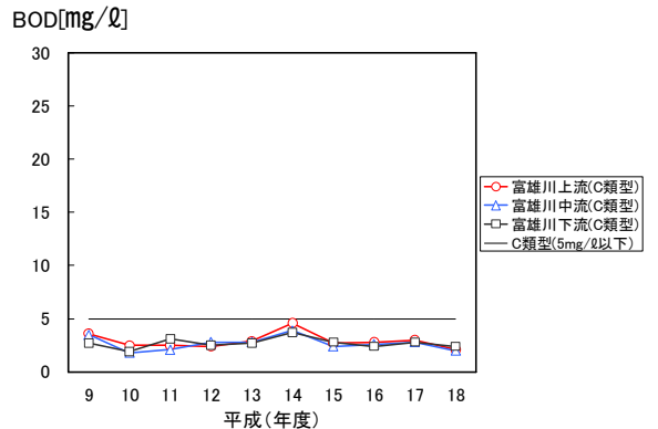
(図-2, 21) 富雄川のBOD推移
