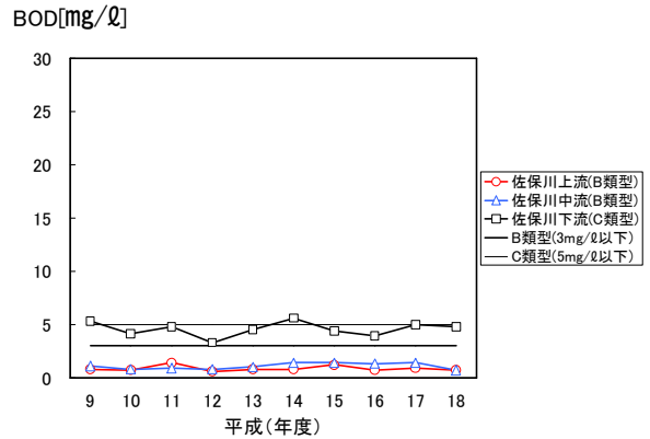
(図-2, 19) 佐保川のBOD推移
