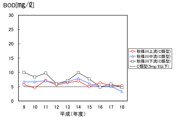
(図-2, 20) 秋篠川のBOD推移
