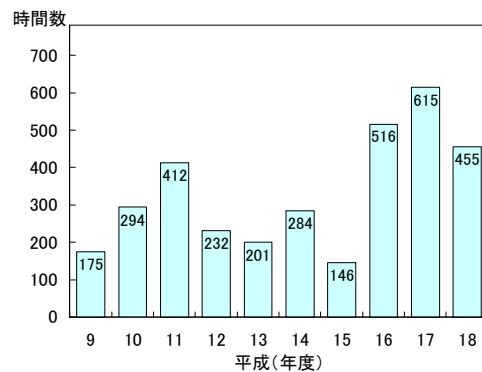
(図-2, 8) 光化学オキシダント (1時間値が0.06ppmを超えた時間数)
