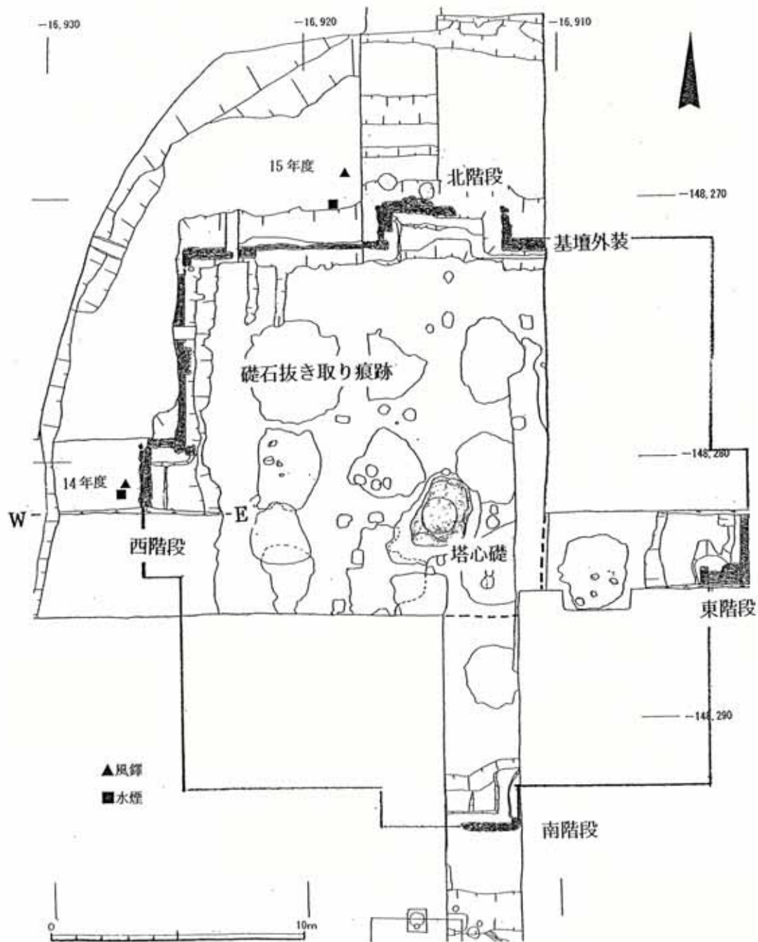
西塔遺構平面図 (S = 1/150)
