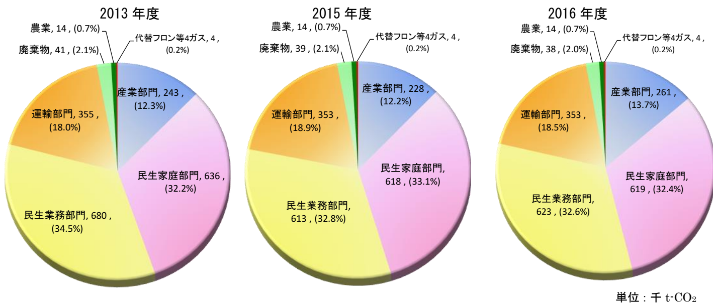
部門別温室効果ガス排出量の推移
