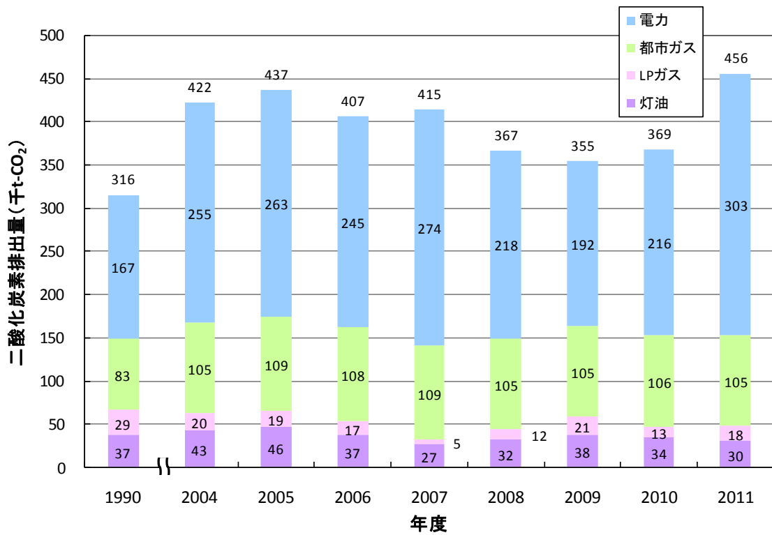
民生家庭部門のエネルギー種別二酸化炭素排出量の推移
