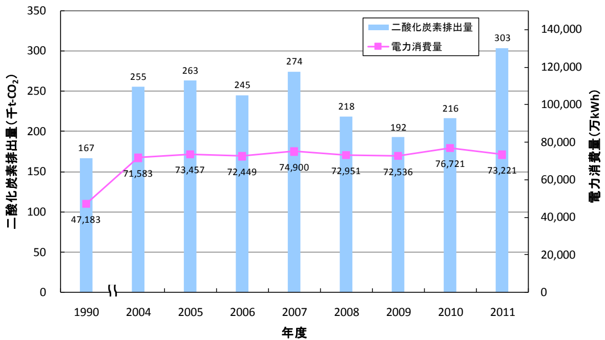
民生家庭部門の二酸化炭素排出量及び電力消費量の推移
