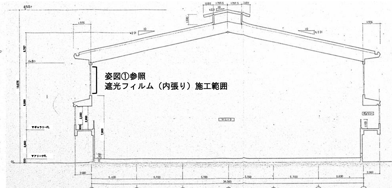
断面図
