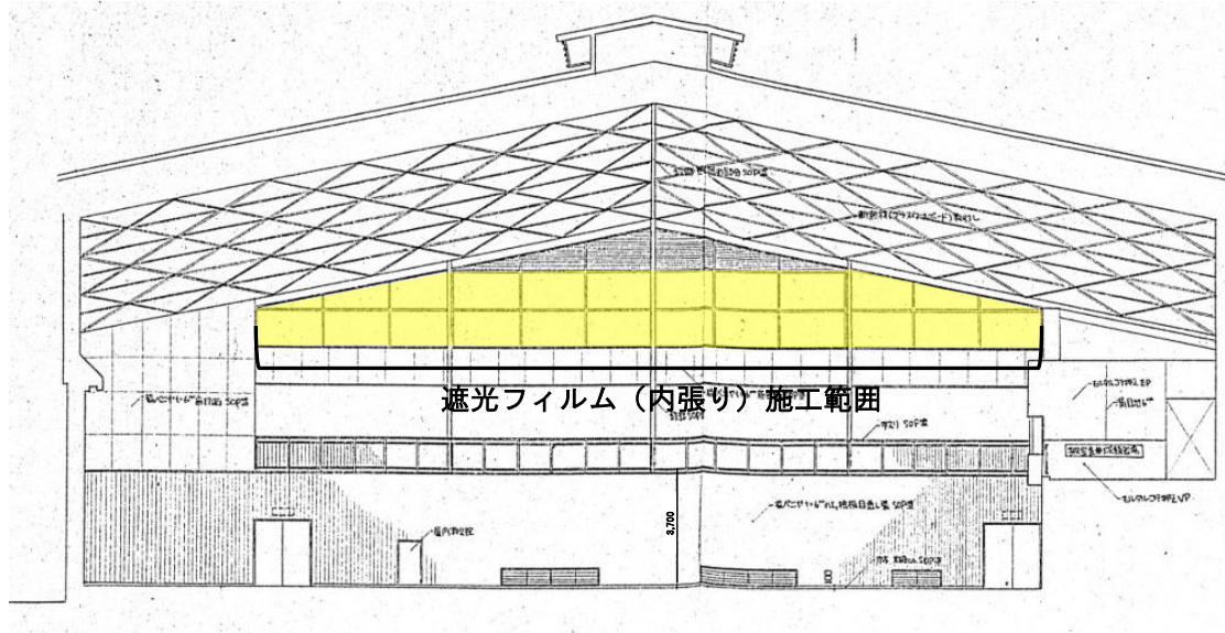
展開図
