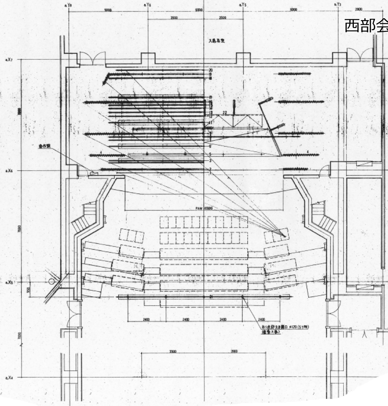
平面図 S=1:50
