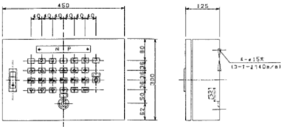
操作盤 S=1:5
