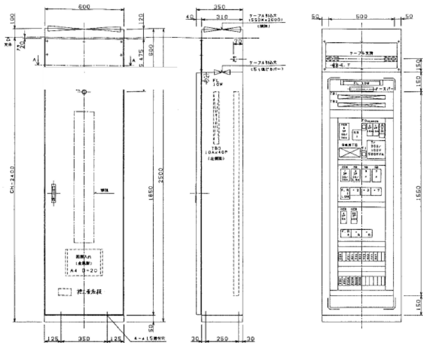
制御盤 S=1:10
