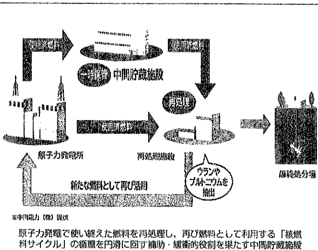
原子力発電で使い終えた燃料を再処理し、再び燃料として利用する「核燃料サイクル」の循環を円滑に回す補助・緩衝的役割を果たす中間貯蔵施設
