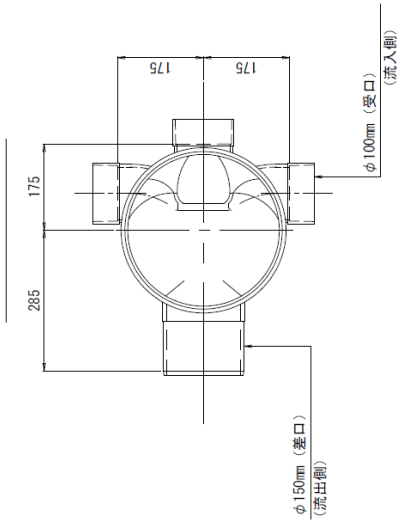
平面図
