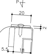
P 矢視図
