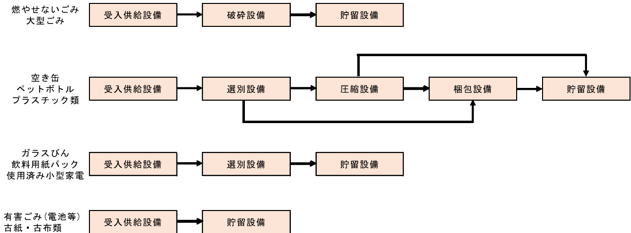
図 13-2 リサイクルセンターの処理フロー
