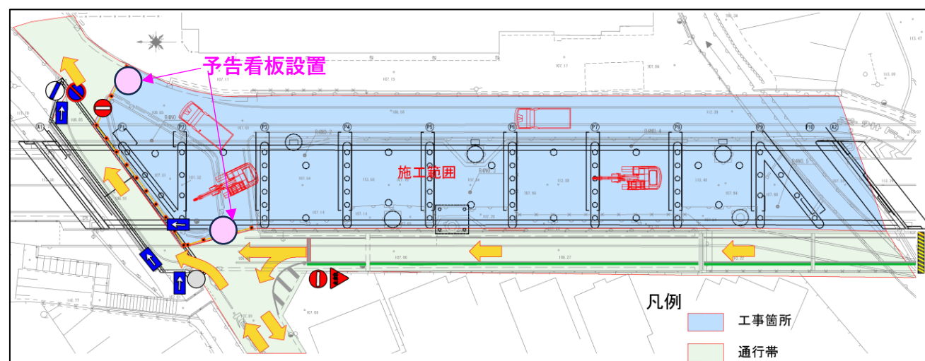
②東側道及び市道309号(西行)通行止め時占用形態（7月上旬～1月中旬）
