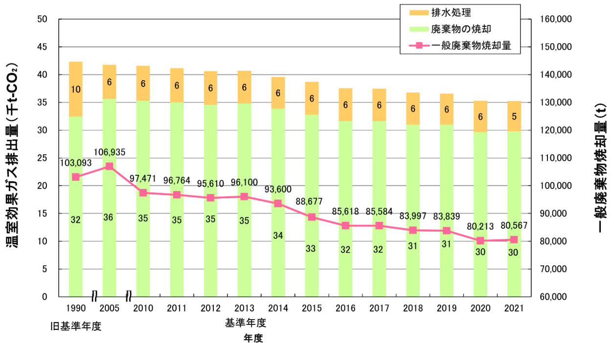
廃棄物分野の系統別温室効果ガス排出量及び一般廃棄物焼却量の推移
