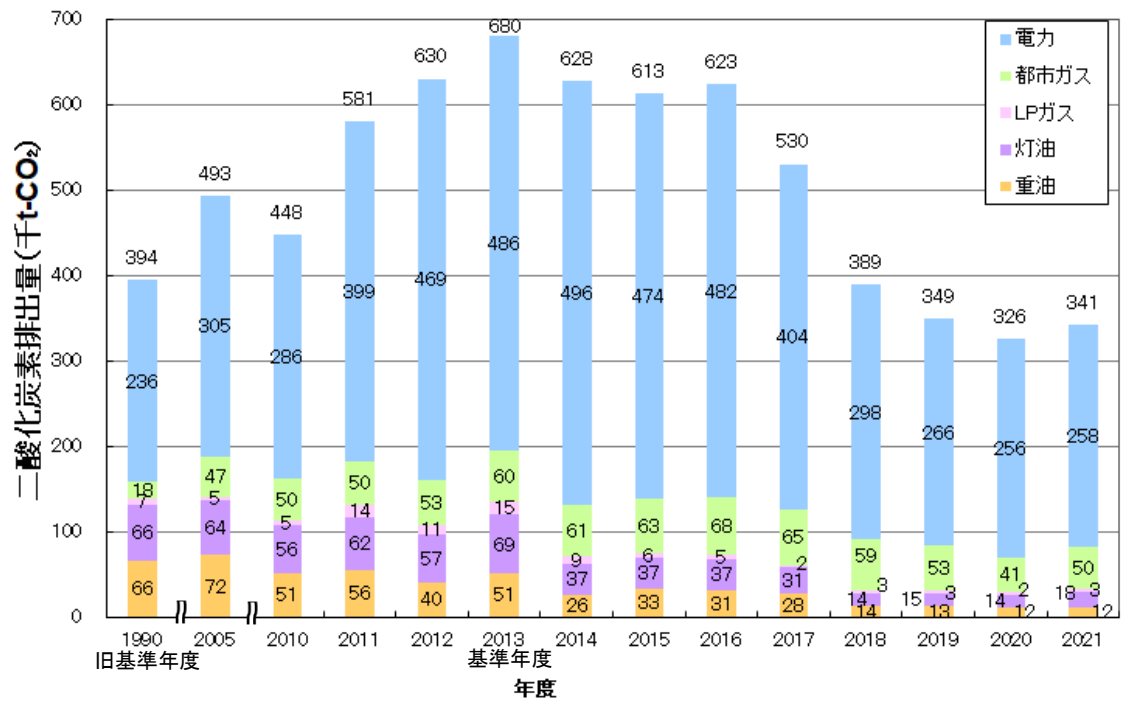
民生業務部門のエネルギー種別二酸化炭素排出量の推移
