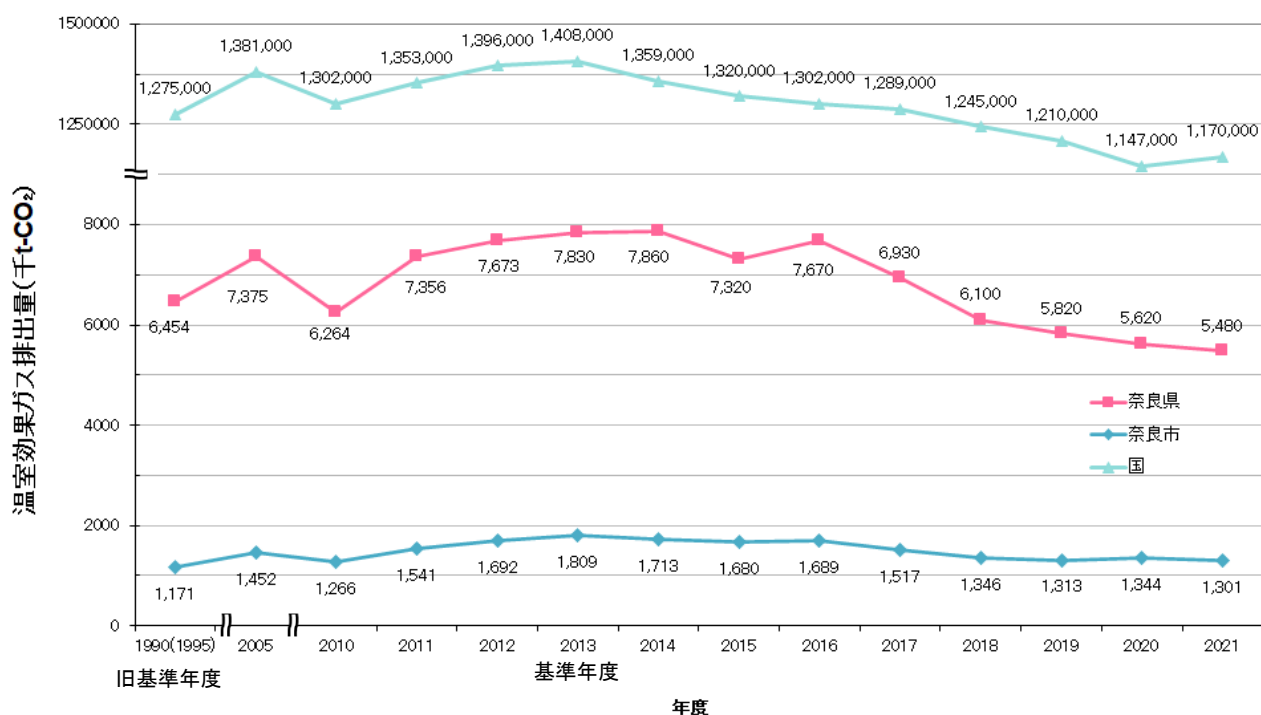
国、奈良県、奈良市の温室効果ガス排出量の推移
