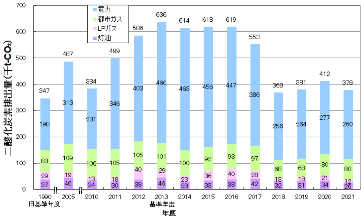
民生家庭部門のエネルギー種別二酸化炭素排出量の推移
