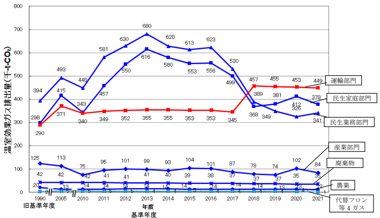
部門別温室効果ガス排出量の推移
