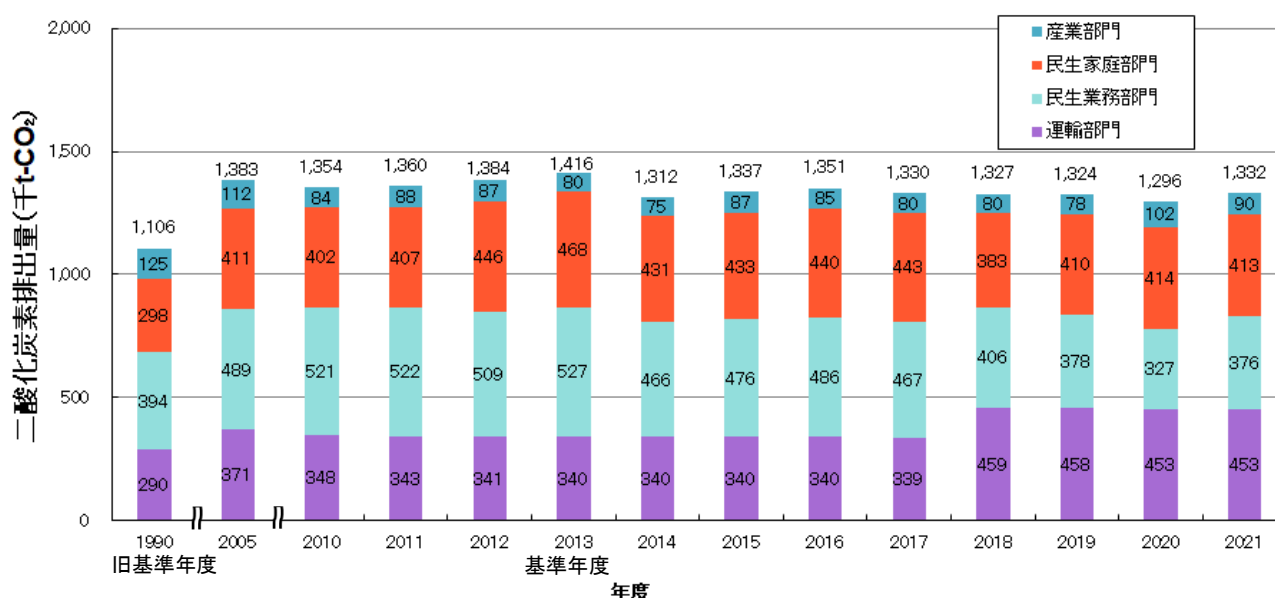
エネルギー起源の二酸化炭素排出量の推移（部門別、係数固定）
