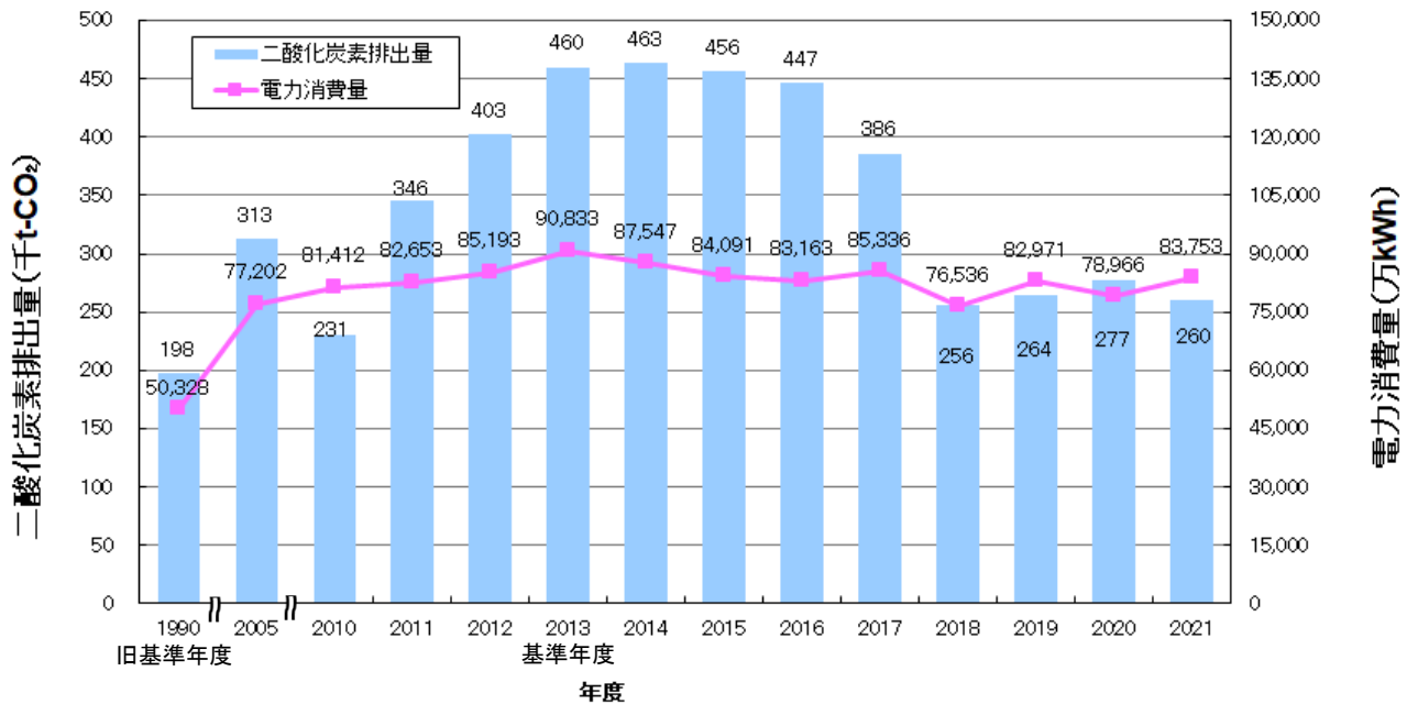
電力由来の二酸化炭素排出量及び電力消費量の推移
