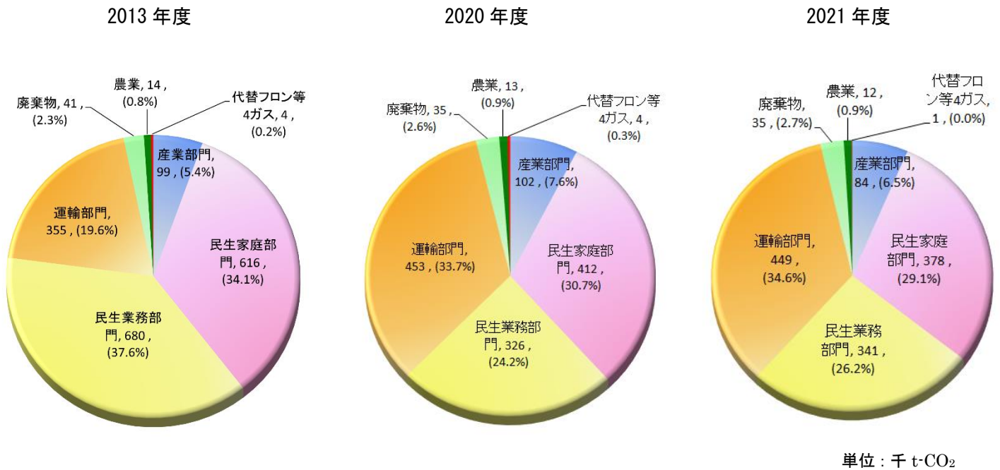
部門別温室効果ガス排出量の推移
