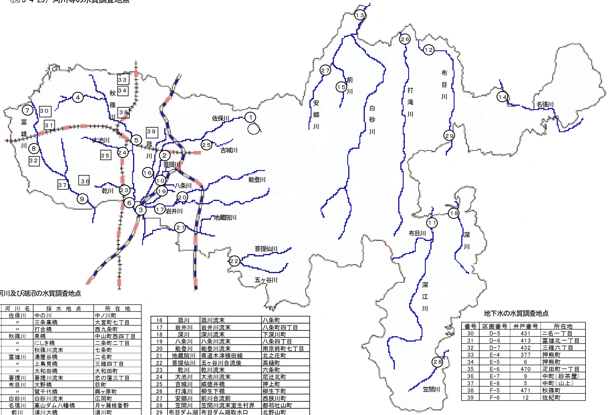
(図 3-4-29) 河川等の水質調査地点
