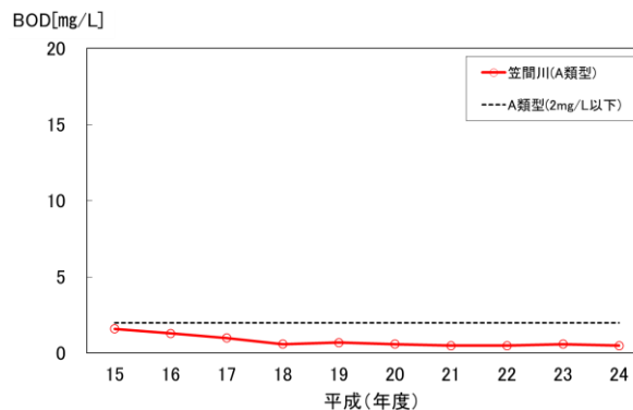
(図3-4-27) 笠間川のBOD推移 (75%値)
