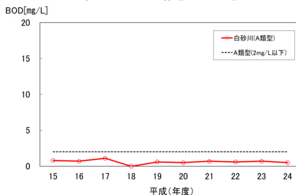
(図3-4-26) 白砂川のBOD推移 (75%値)
