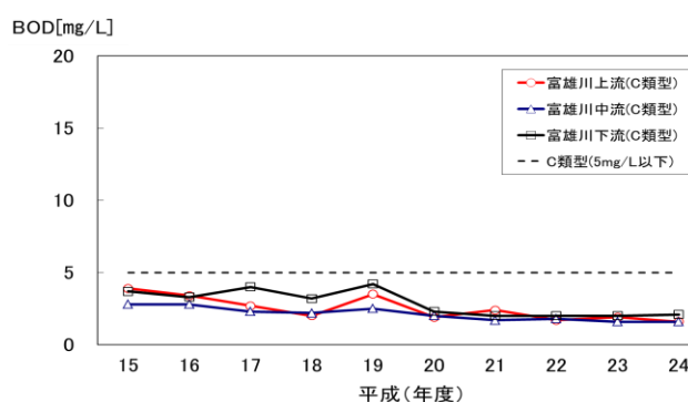
(図3-4-23) 富雄川のBOD推移 (75%値)
