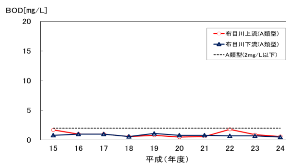
(図3-4-25) 布目川のBOD推移 (75%値)
