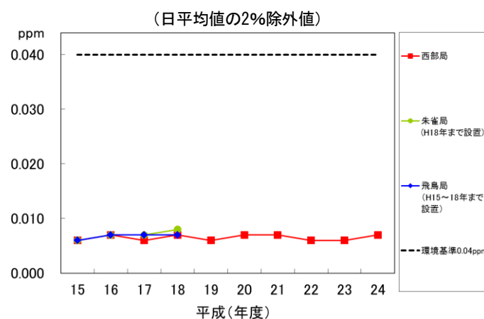
(図3-4-2) 二酸化硫黄 長期的評価の経年変化
