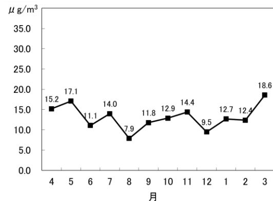
(図3-4-12) 微小粒子状物質濃度の月平均値 (平成24年度)
