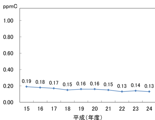
(図3-4-13) 非メタン炭化水素濃度の 経年変化 (年平均値)
