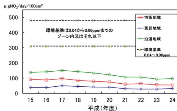
(図3-4-17) 二酸化窒素の経年変化
