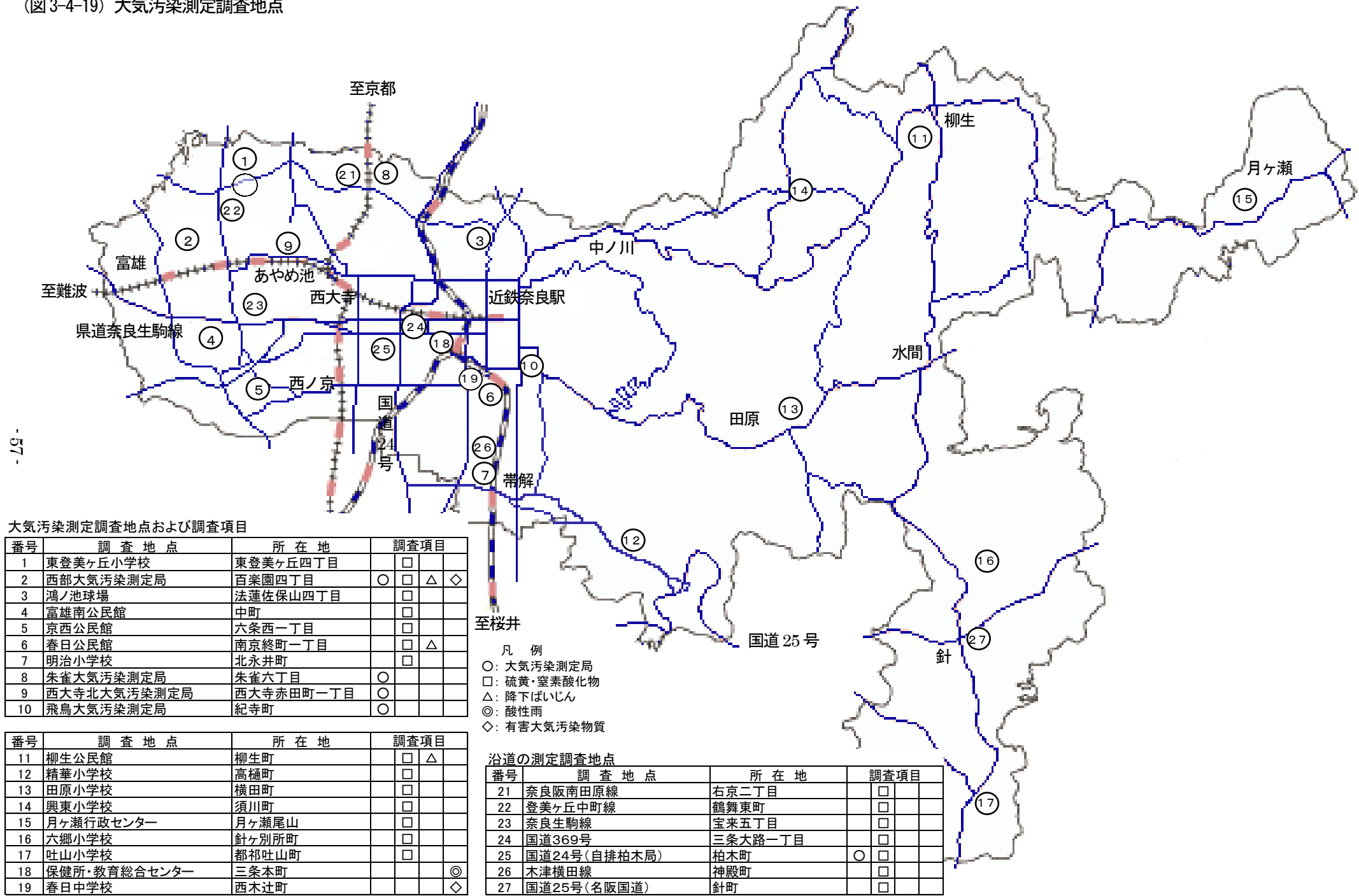
(図 3-4-19) 大気汚染測定調査地点
