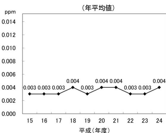
(図3-4-1) 二酸化硫黄濃度の経年変化
