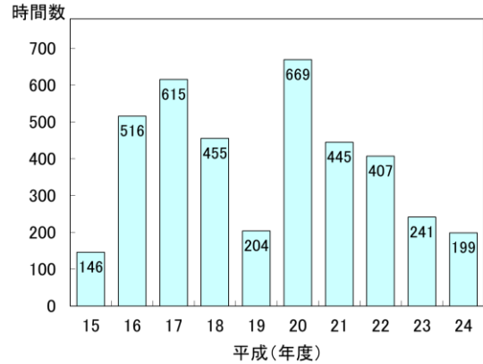
(図3-4-8) 光化学オキシダント (1時間値が0.06ppmを超えた時間数)
