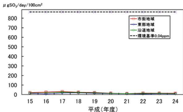
(図3-4-16) 硫黄酸化物の経年変化
