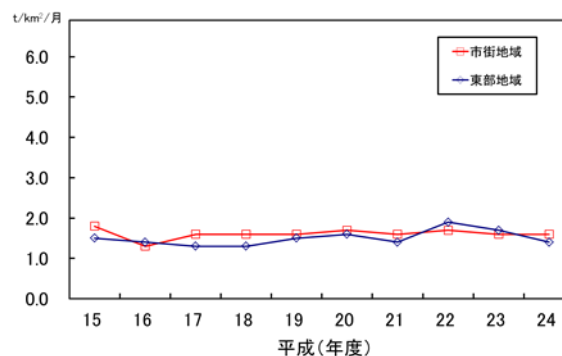
(図3-4-15) 降下ばいじんの経年変化
