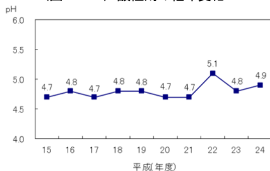
(図3-4-18) 酸性雨の経年変化
