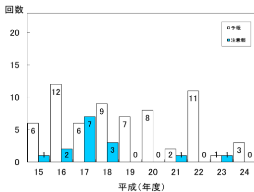
(図3-4-9) 光化学スモッグ発令回数の 経年変化
