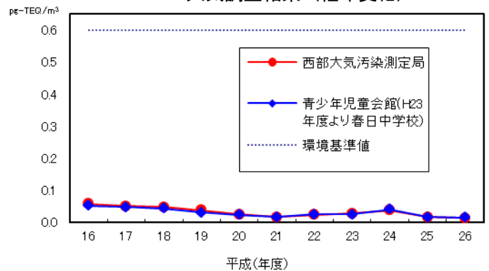
(図3-4-30) ダイオキシン類の大気調査結果 (経年変化)
