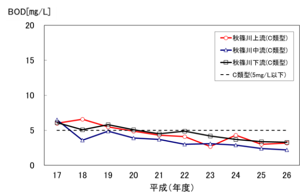
(図3-4-21) 秋篠川のBOD推移 (75%値)
