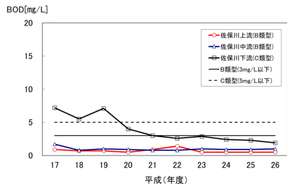
(図3-4-20) 佐保川のBOD推移 (75%値)
