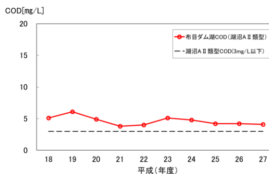
(図3-4-25) 布目ダム湖のCOD推移（75%値）
