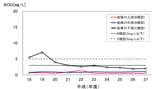
(図3-4-18) 佐保川のBOD推移（75%値）
