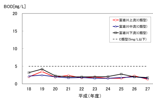
(図3-4-20) 富雄川のBOD推移（75%値）
