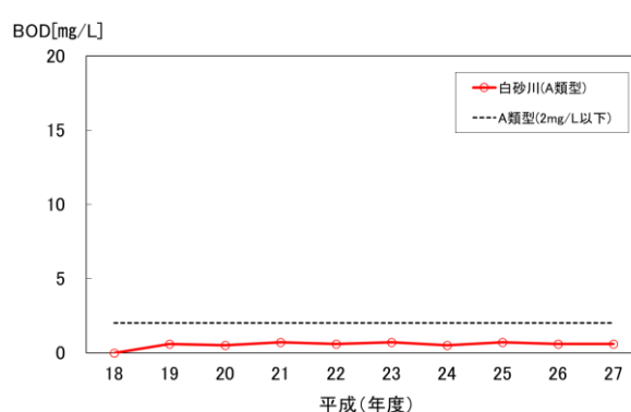
(図3-4-23) 白砂川のBOD推移 (75%値)
