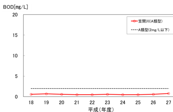
(図3-4-24) 笠間川のBOD推移 (75%値)
