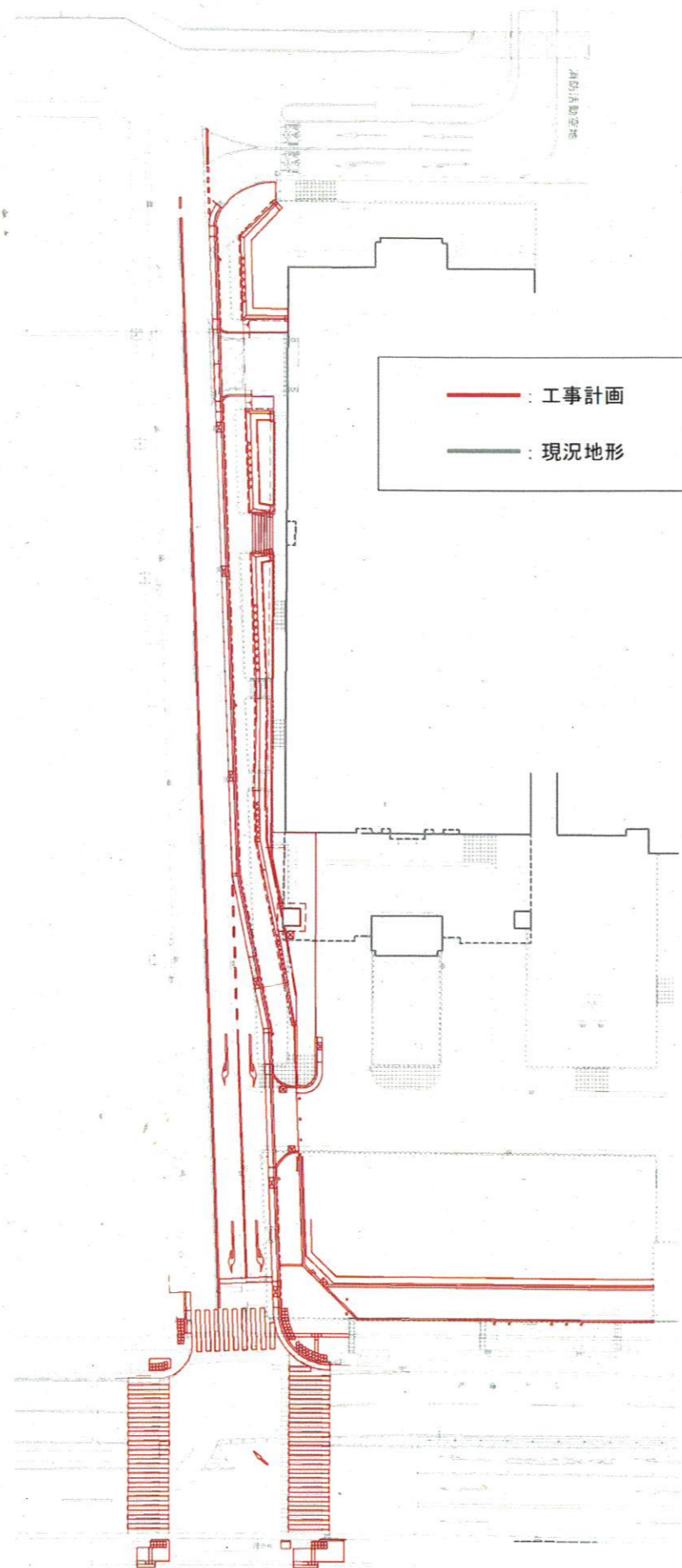
工事概要図
