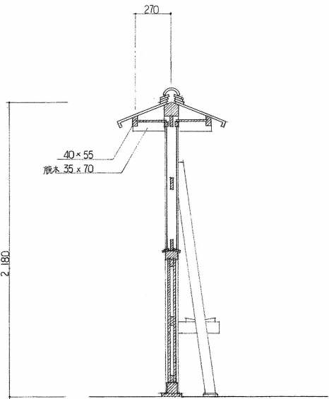
矩計図
