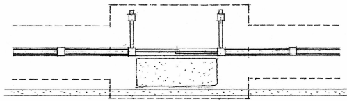
平面図
