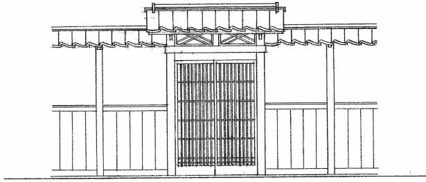
立面図
