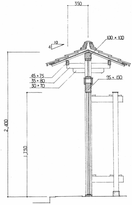
矩計図
