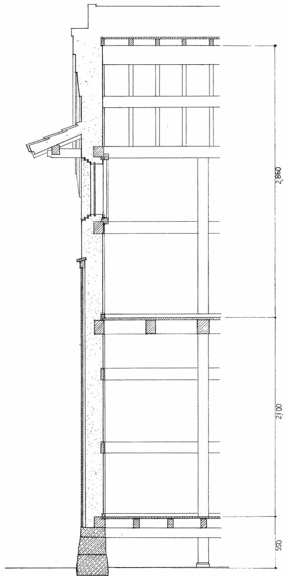
矩計図
