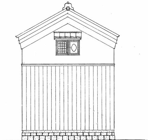
トオリに妻を見せた立面図
