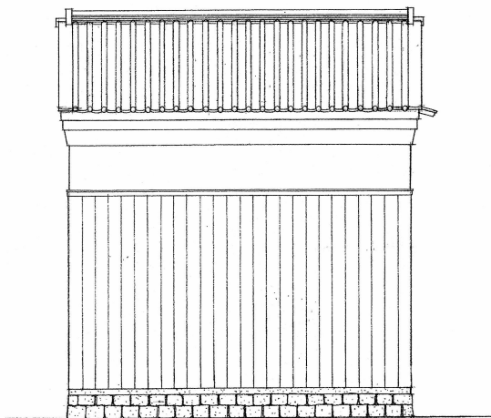
トオリに平を見せた立面図
