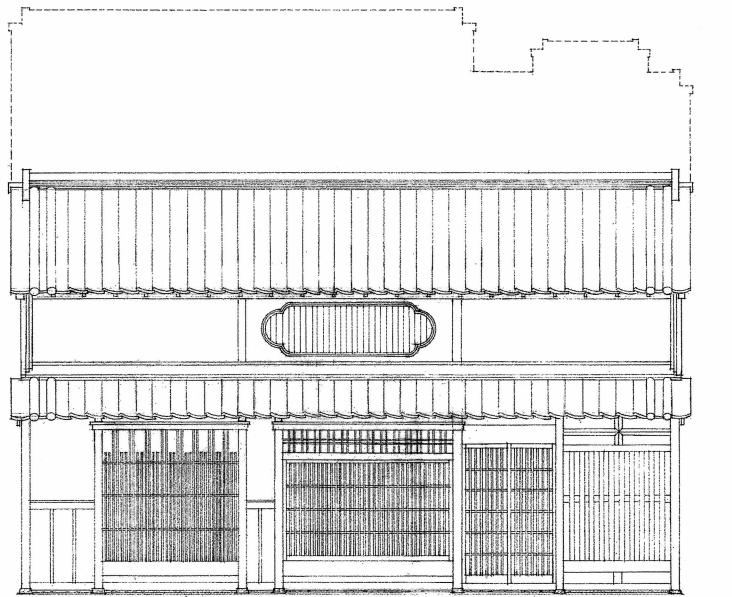
立面図
