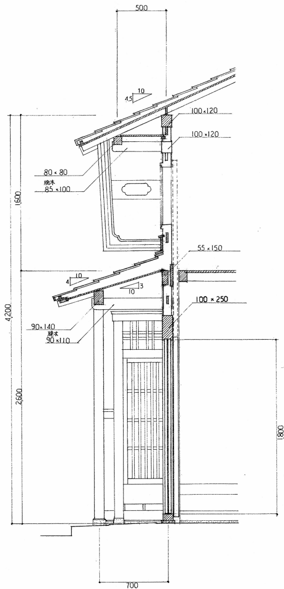
矩計図
