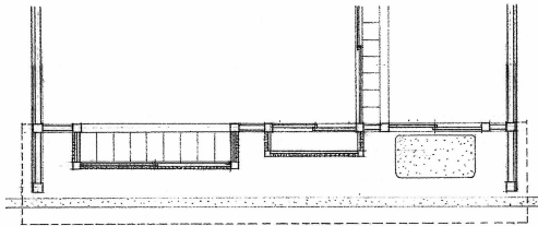
1階平面図
