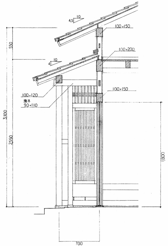
矩計図
