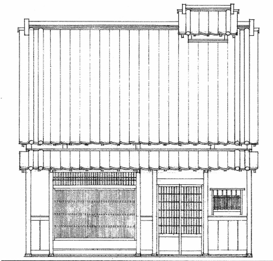
立面図
