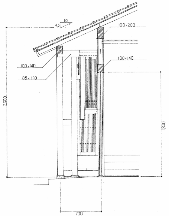
矩計図
