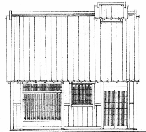
立面図
