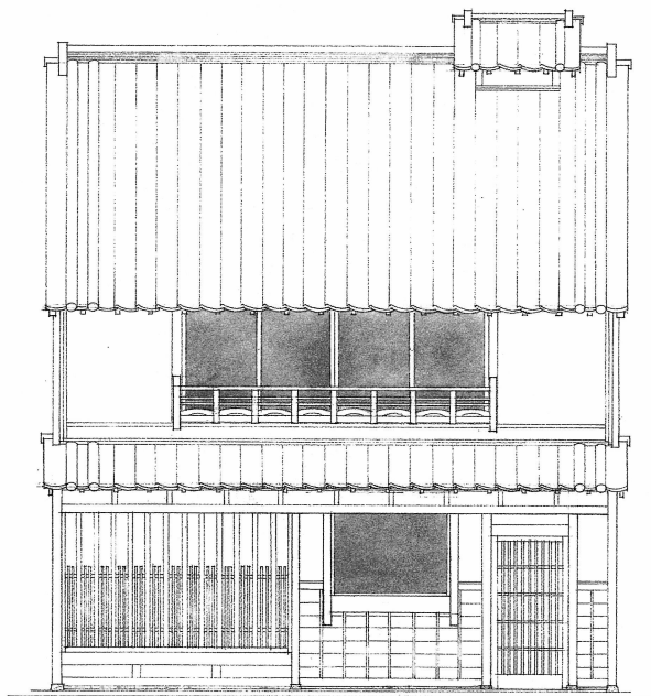
立面図
