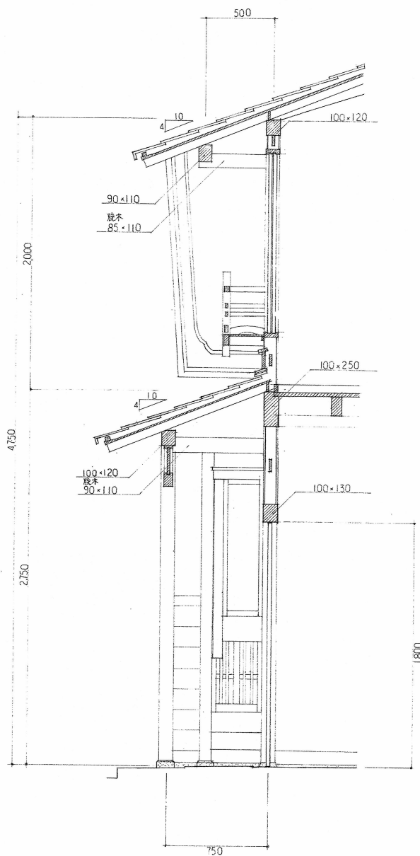
矩計図
