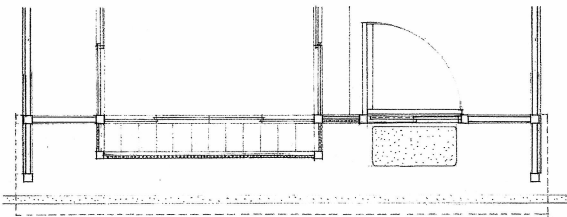
1階平面図
