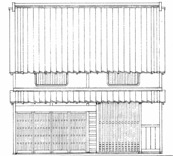
立面図
