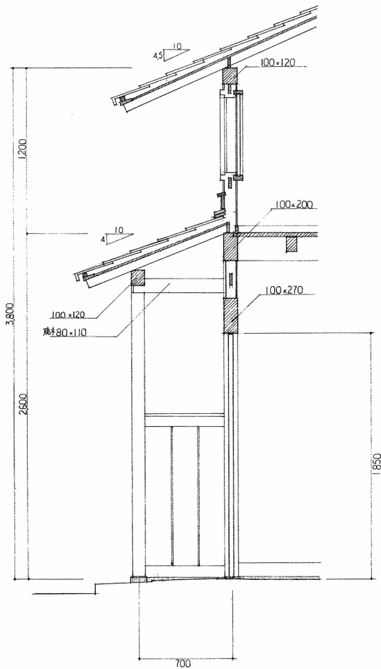
矩計図
