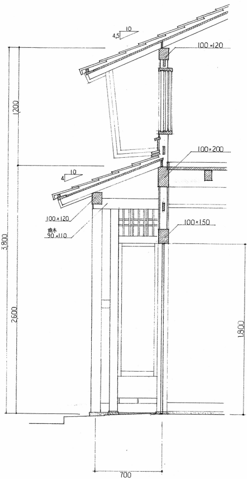
矩計図
