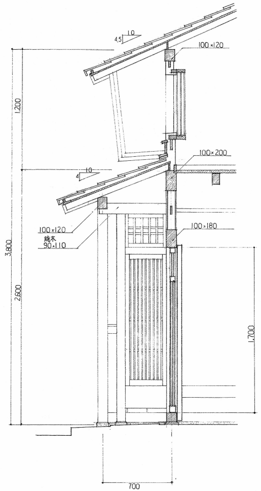
矩計図
