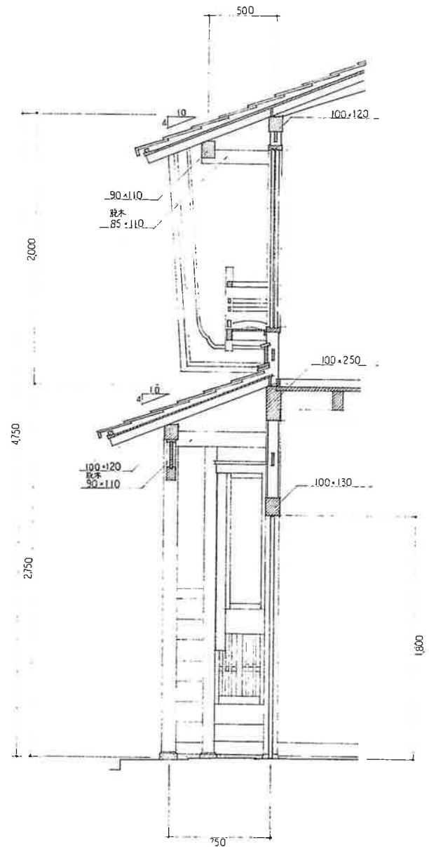
矩計図
