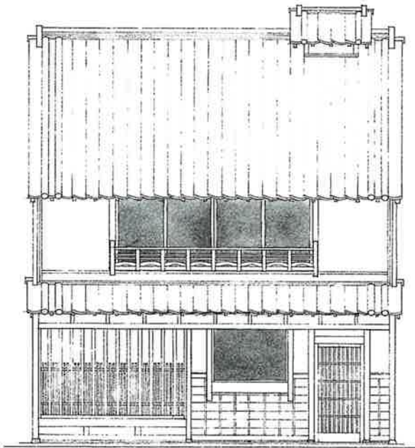
立面図
