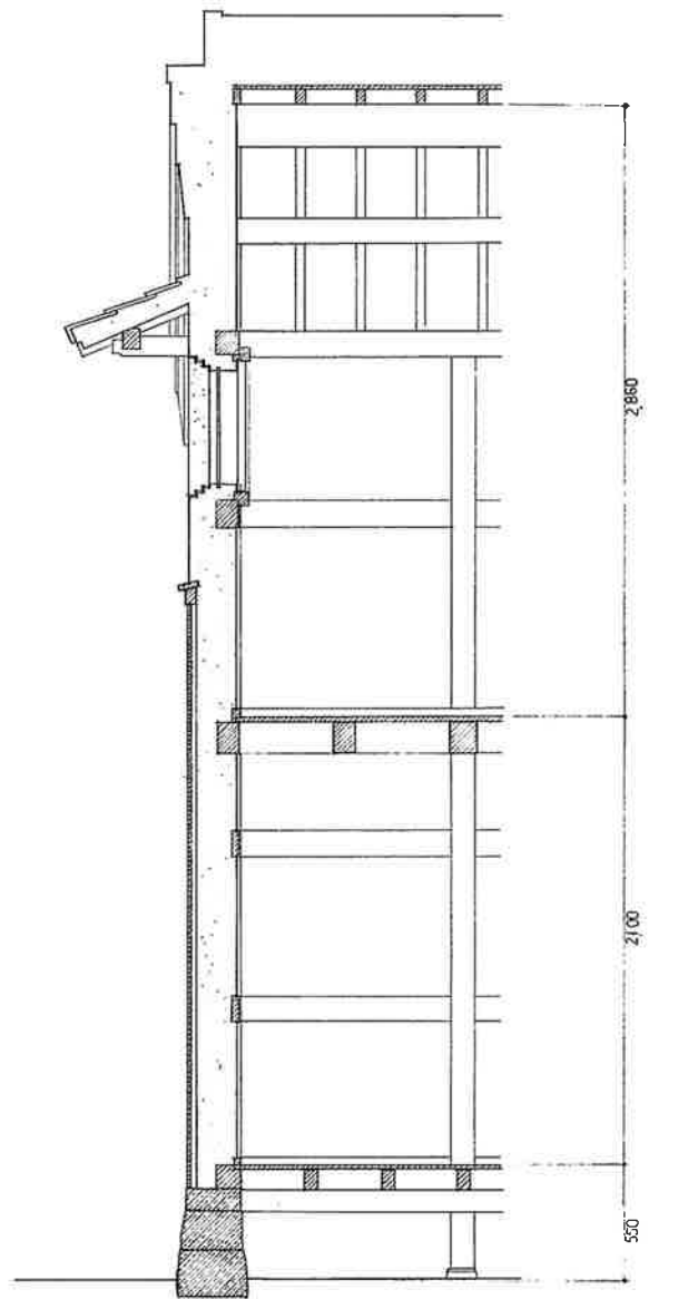
矩計図
