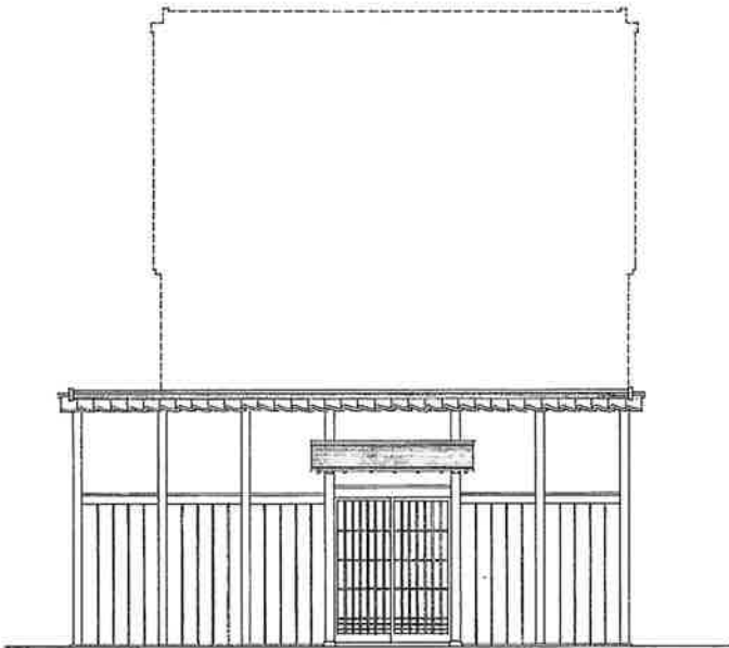
立面图
