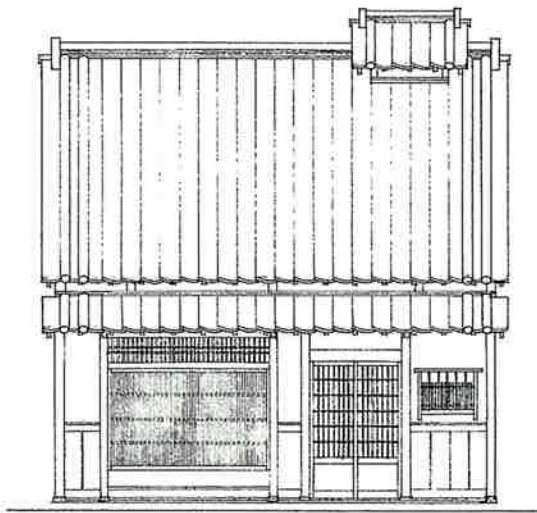
立面図
