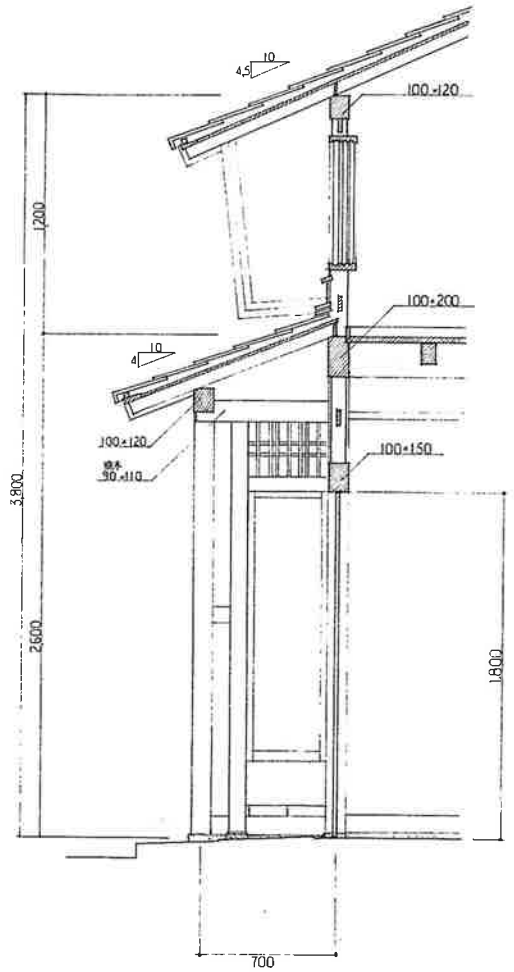
矩計図
