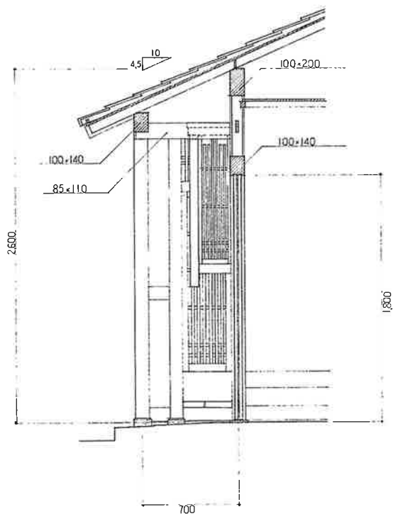
矩計図
