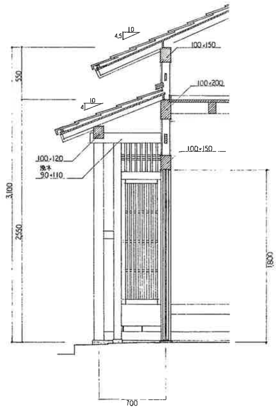
矩計図
