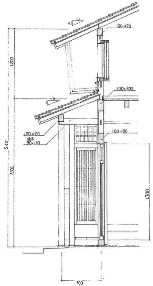
矩計図
