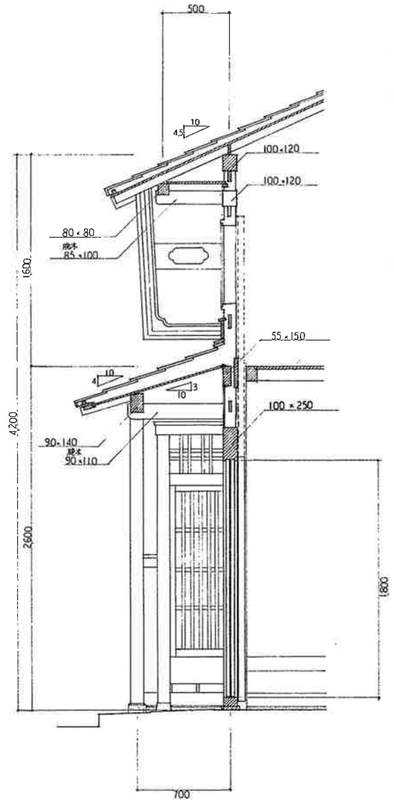
矩計図
