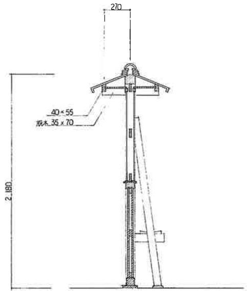
矩計図
