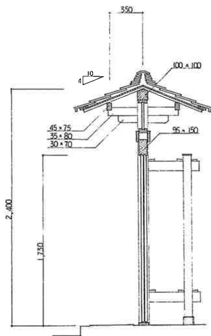
矩計図
