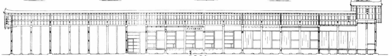
南側から見た断面図
