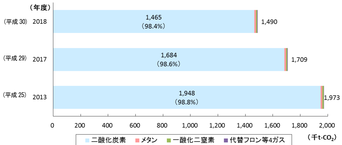
(図 2-1-1) 種類別温室効果ガス排出量
