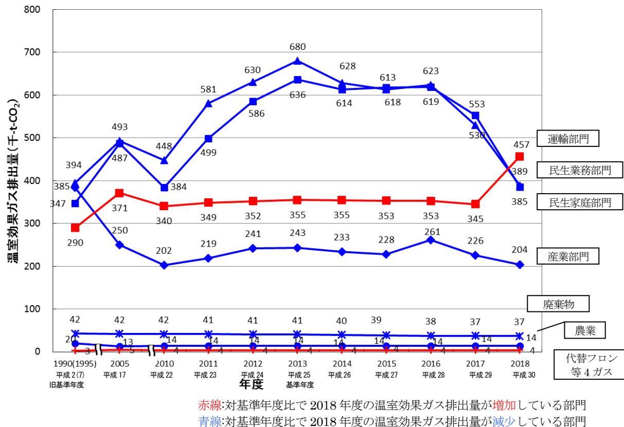
（図 2-1-4）部門別温室効果ガス排出量の推移
