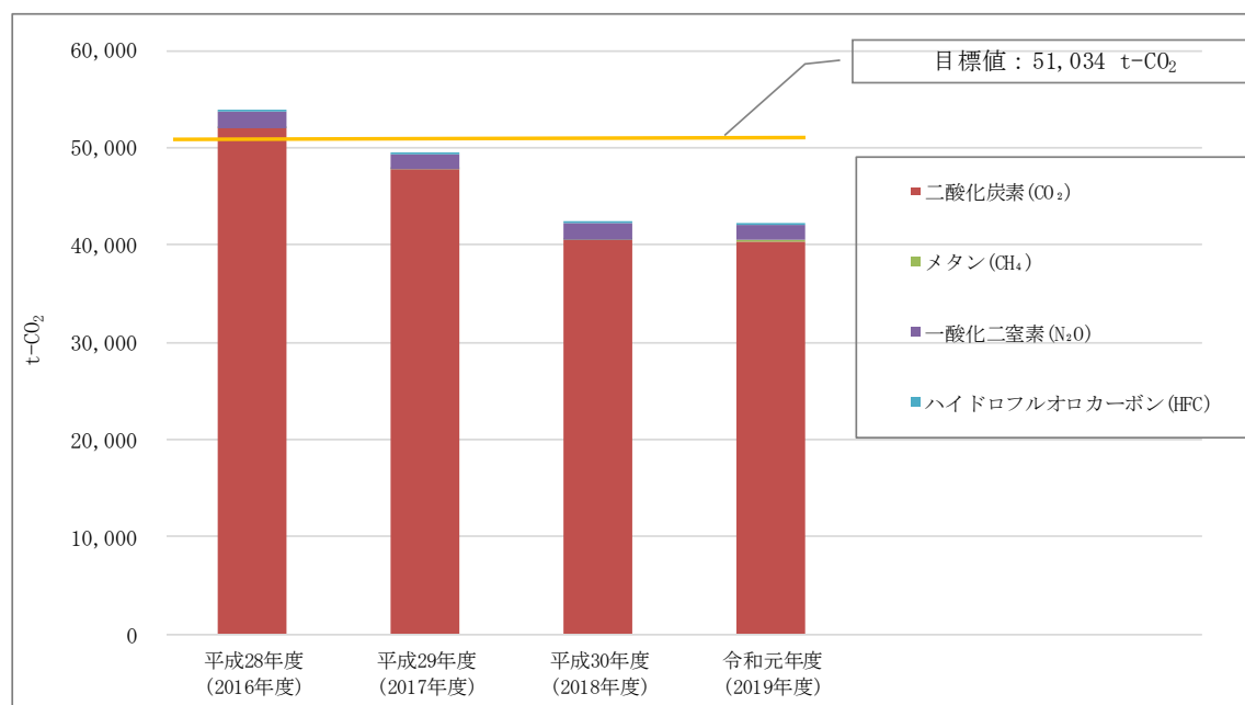
(図 2-1-6) 温室効果ガス排出量推移
