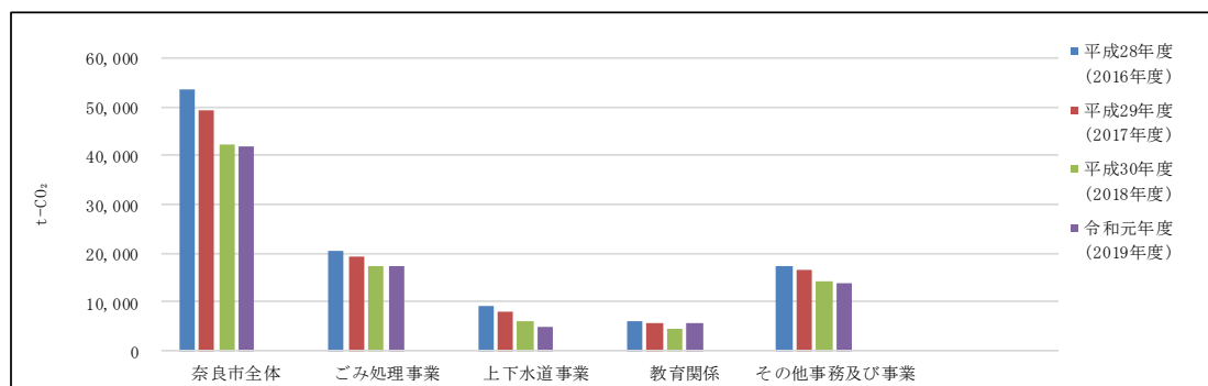
(図 2-1-8) 事業別温室効果ガス排出量推移
