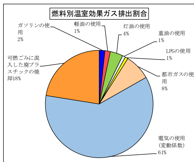
(図 2-1-7) 燃料別温室効果ガス排出割合
