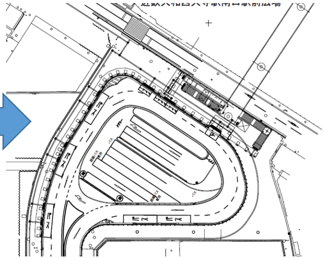
近鉄大和西大寺駅南口駅前広場（令和 3 年 3 月完成）
