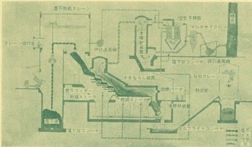
ジンカイ焼却炉系統図
