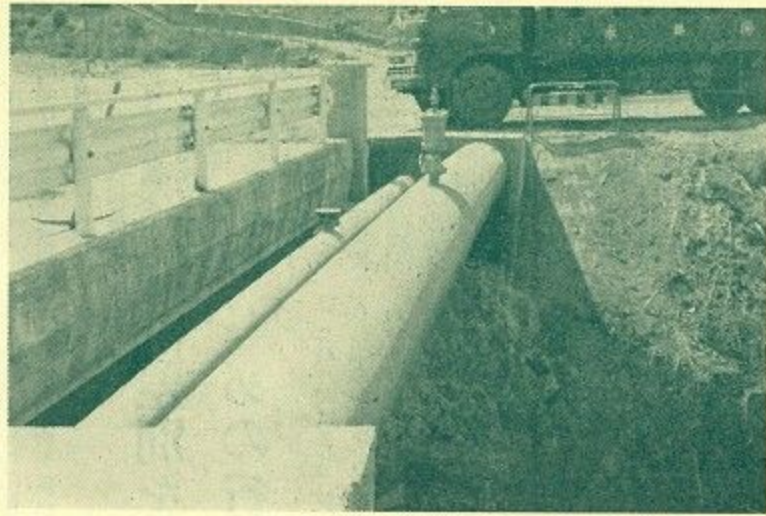
完成した口径700 mm の水管橋 (天理市岩屋町の高瀬川で)
