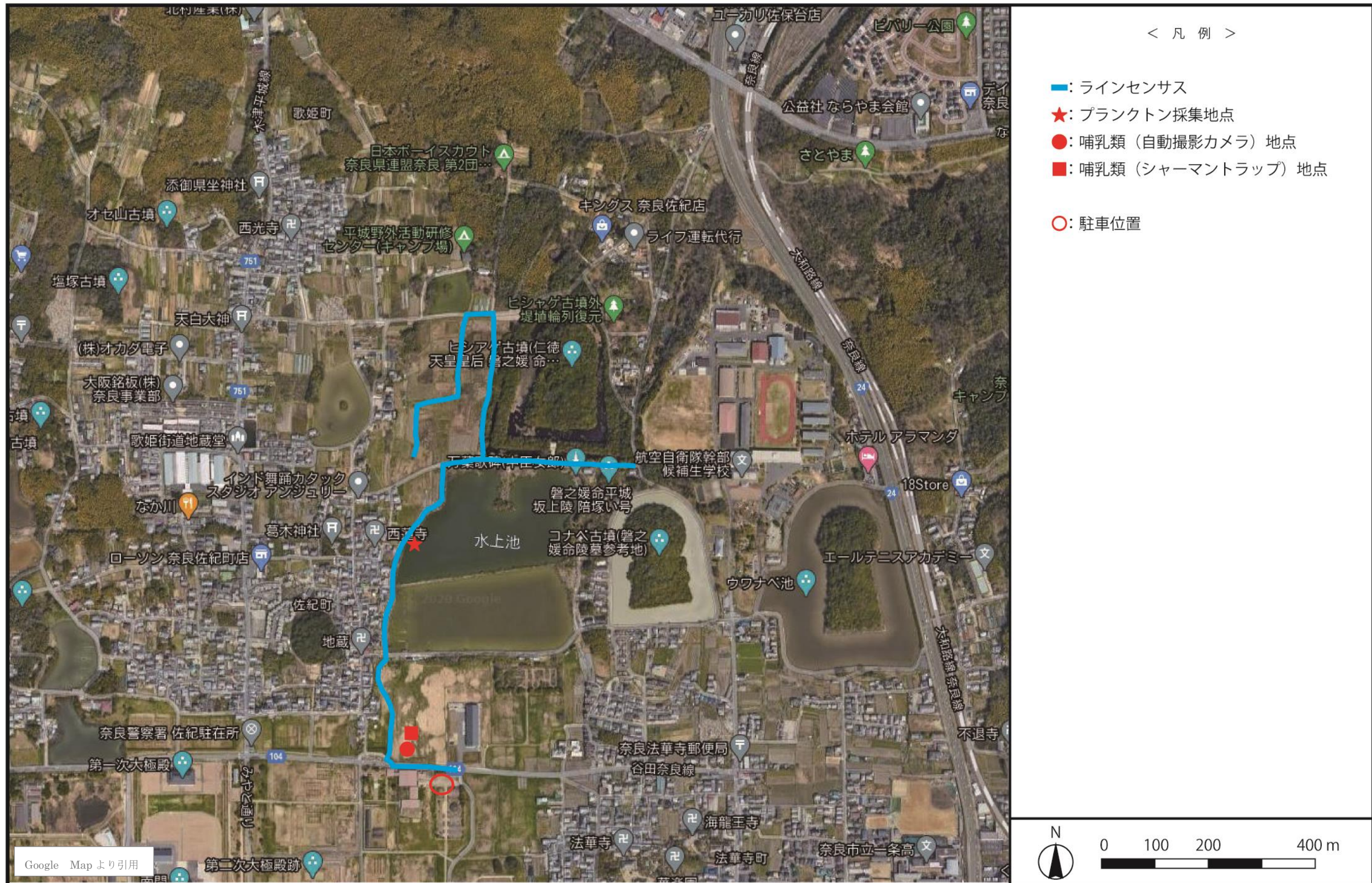
図5 佐紀エリアの調査地点
