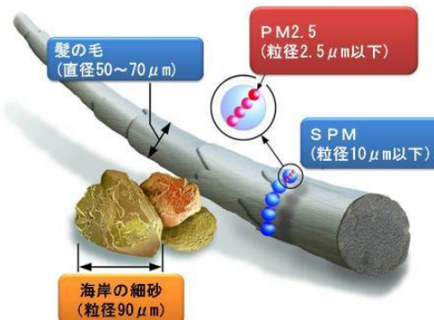
ぴーえむ おお がいけんず PM2.5の大きさ(概念図) しゅつてん しりょう (出典: USEPA資料)
