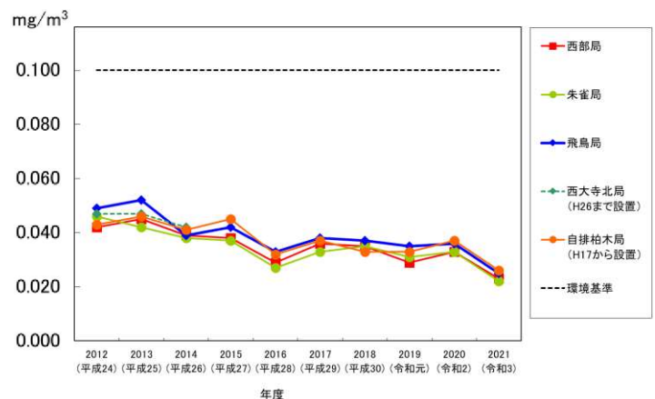
(図3-4-9) 浮遊粒子状物質 長期的評価の経年変化 (日平均値の2%除外値)
